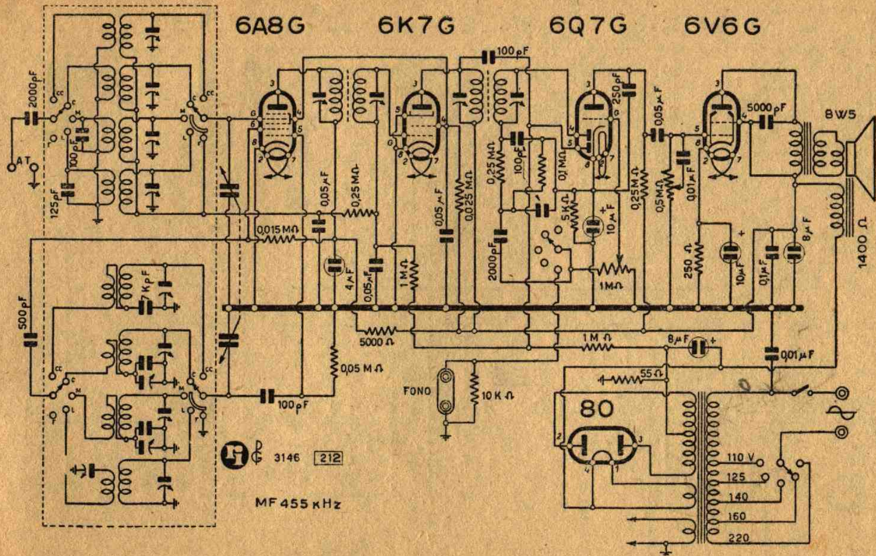
Lo schema elettrico del mod. 411 Siare
